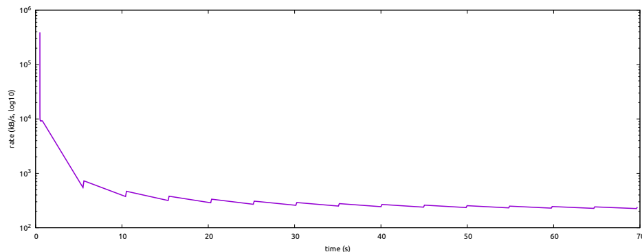
FIGURA 17.4: Tasa de envío medida en el emisor (promedio acumulado)
