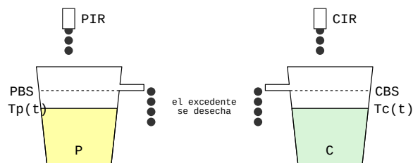
FIGURA 17.13: Algoritmo de cubo de tokens de tipo trTCM
